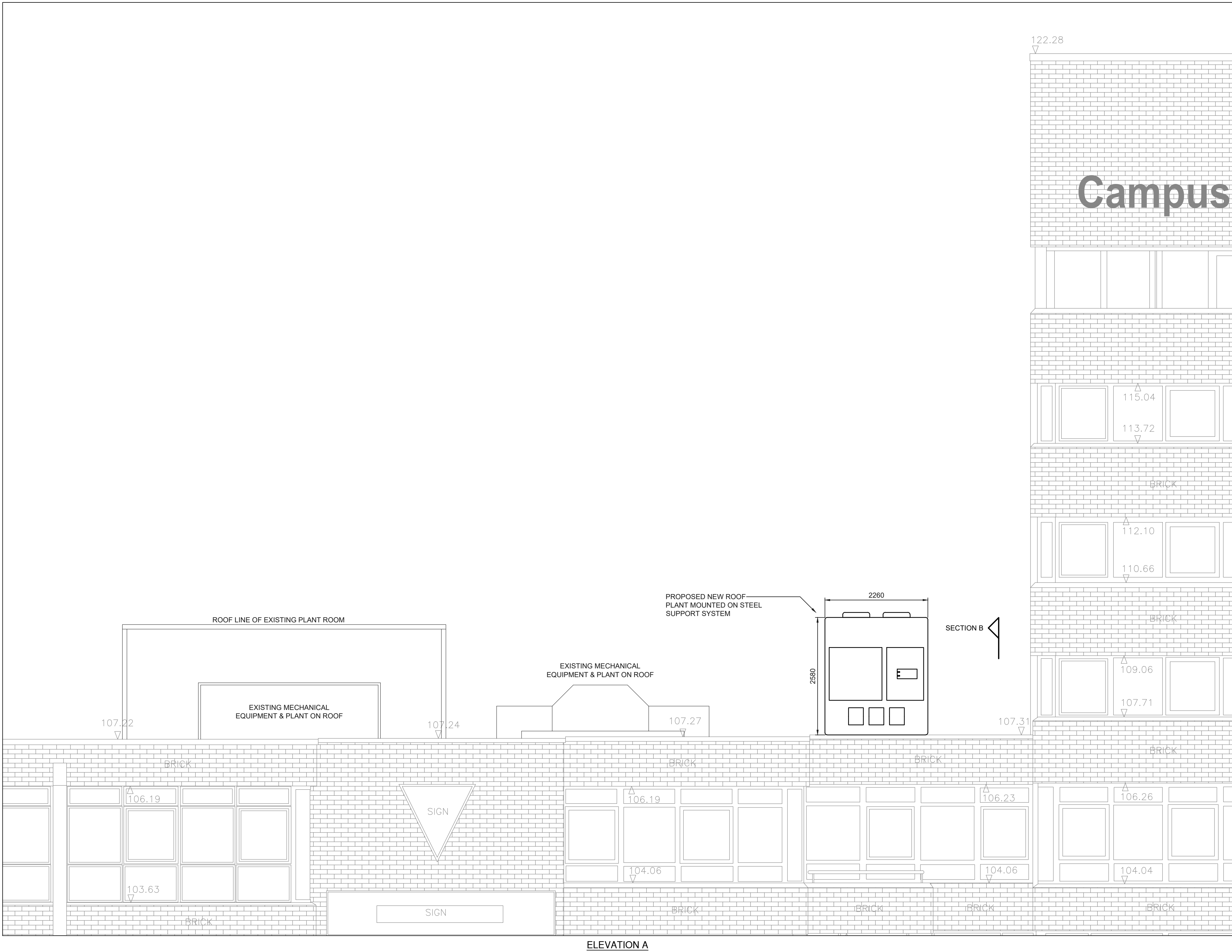
ELEVATION A
