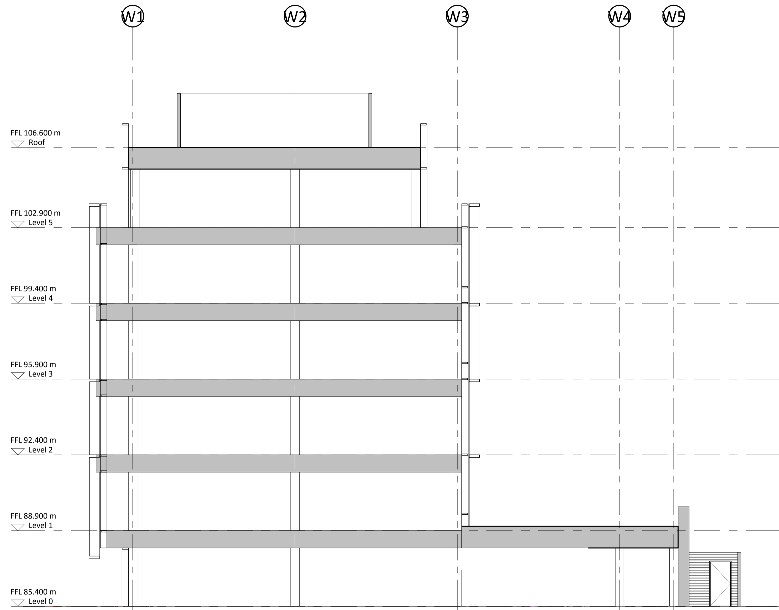
1 Section AA 1 : 100
