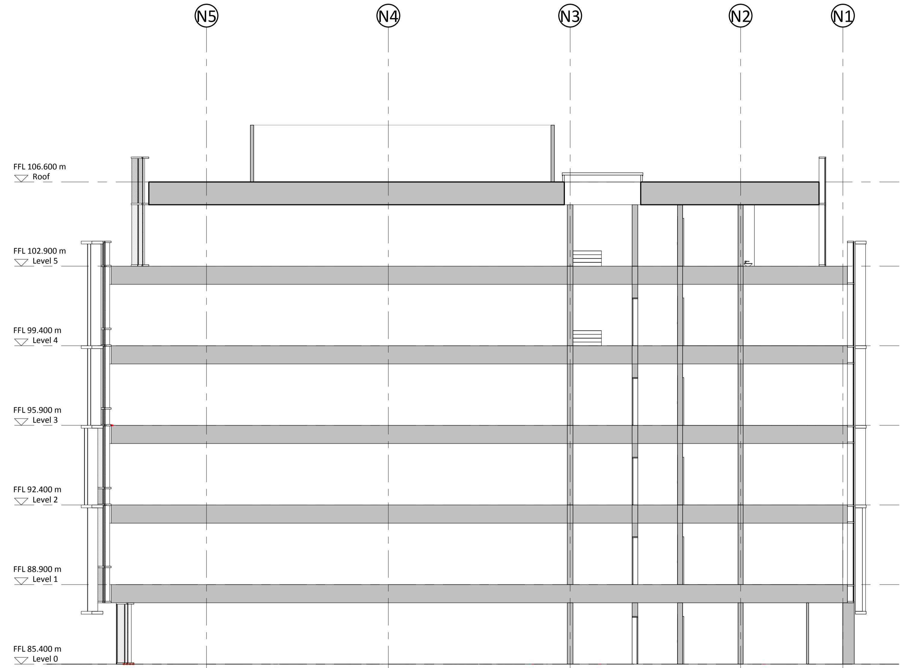
2 Section BB 1 : 100
