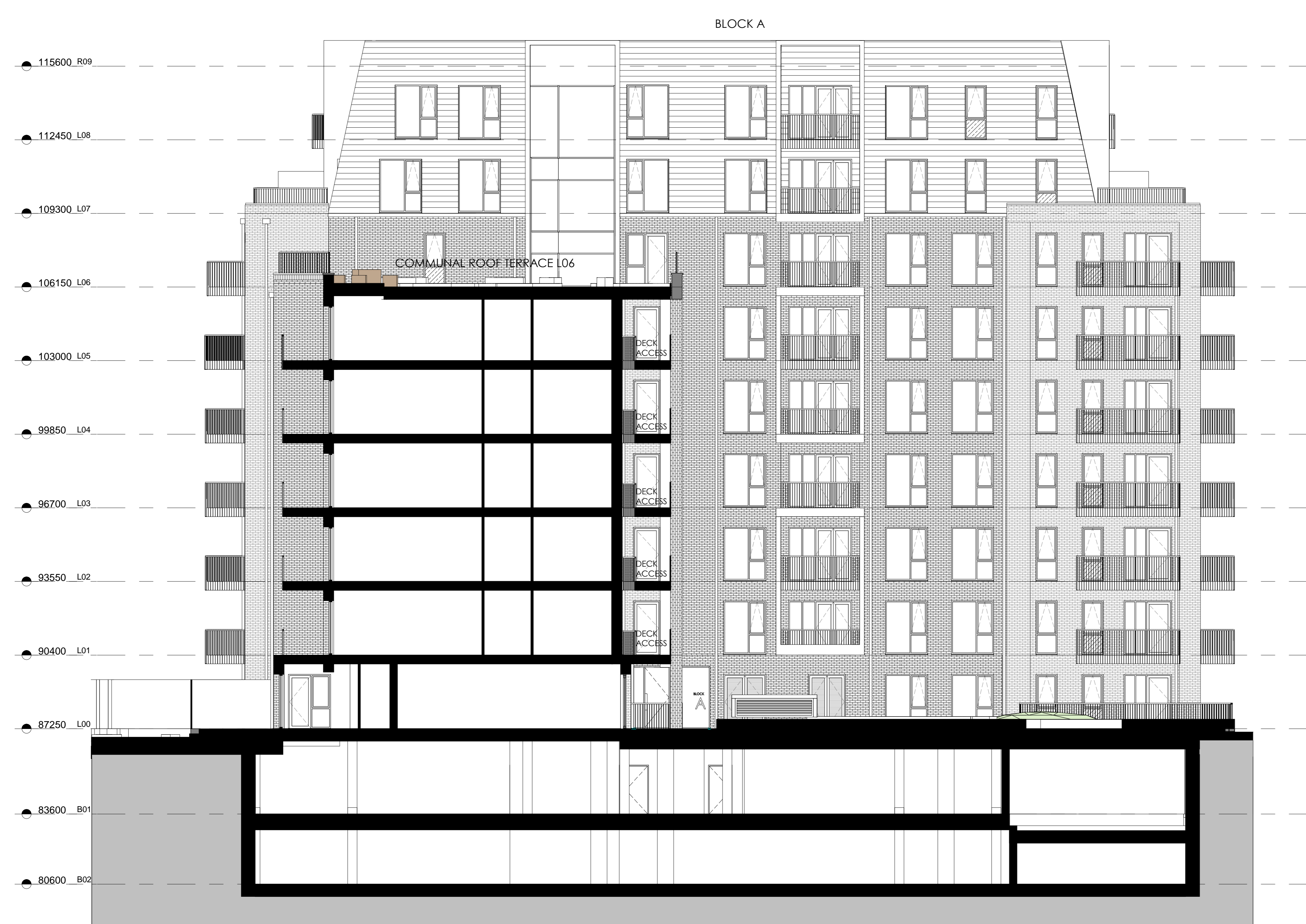
1 Section C 1 : 100
