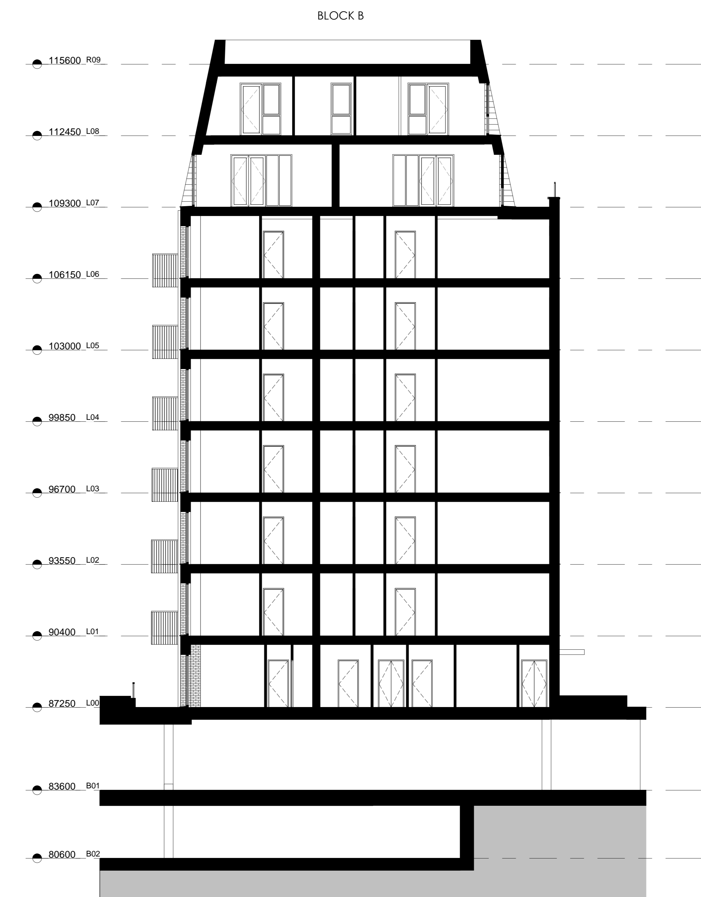
2 Section D 1 : 100
