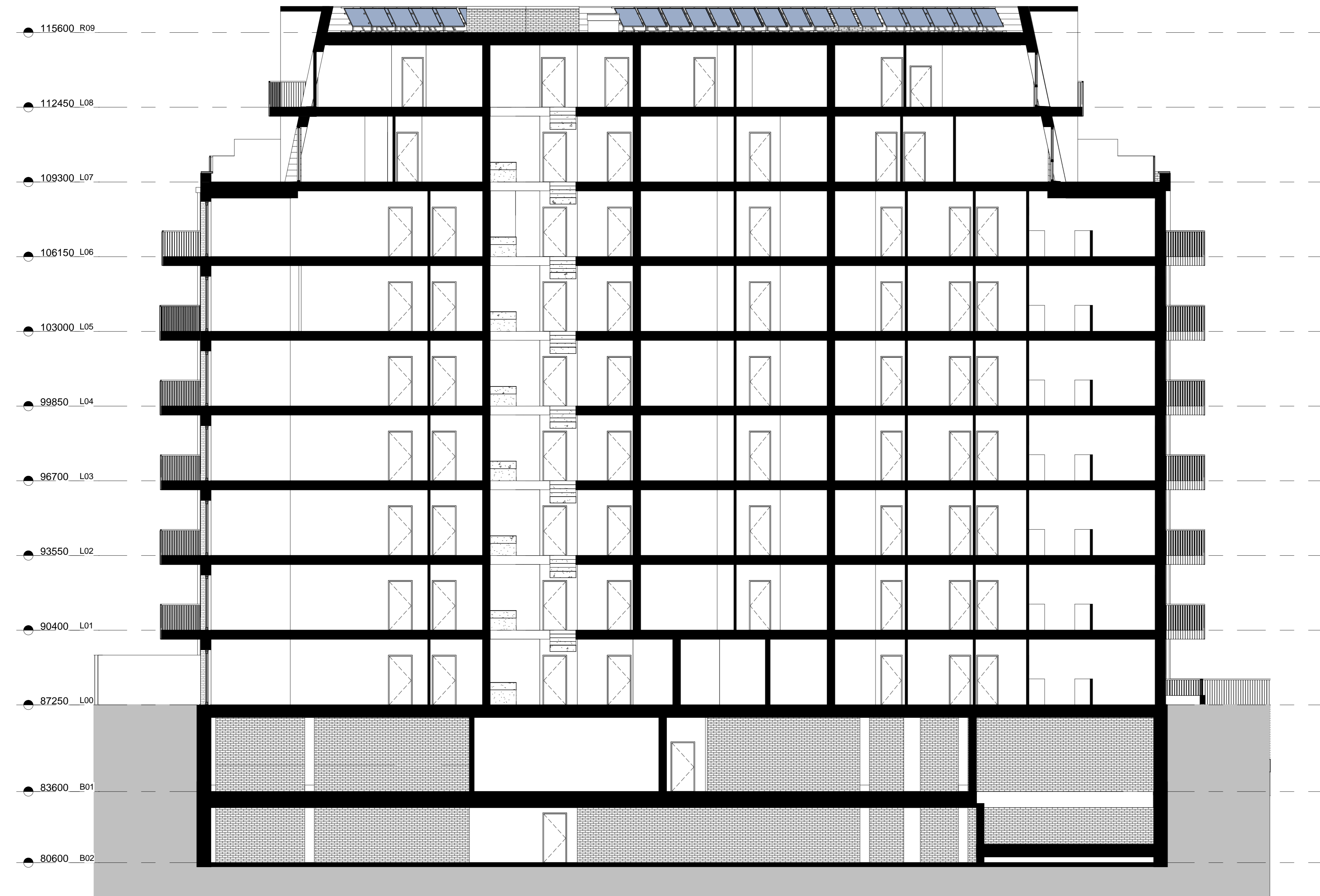
2 Section B 1 : 100
