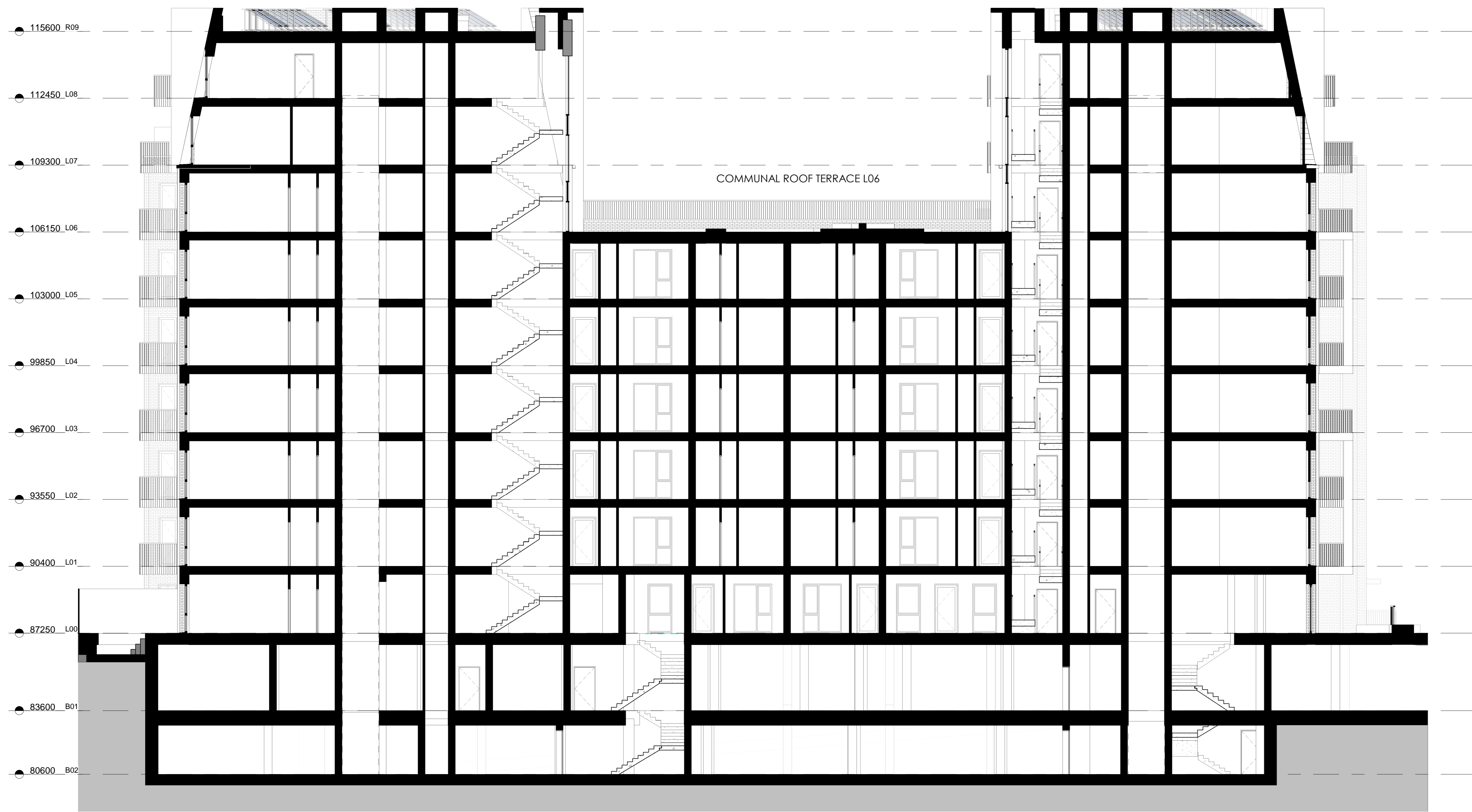
1 Section A 1 : 100
