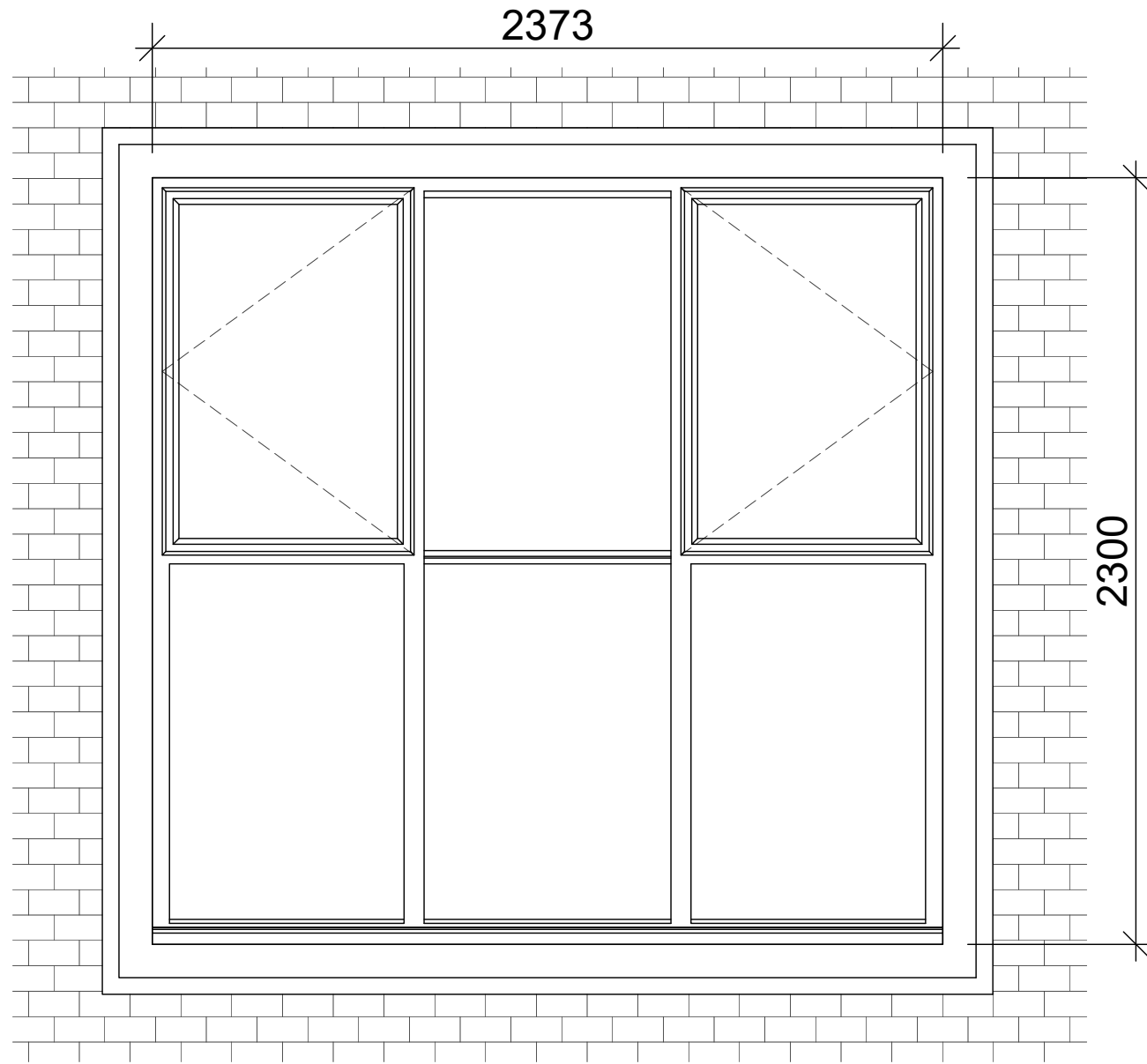
ELEVATION 1 : 20
