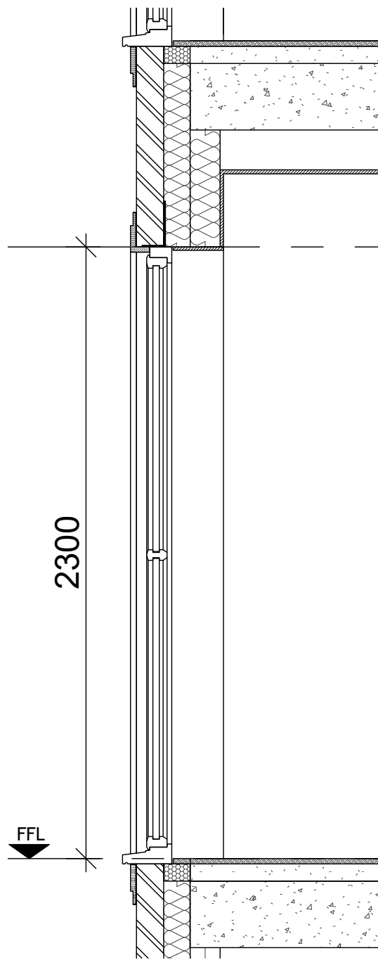
SECTION 1 : 20
