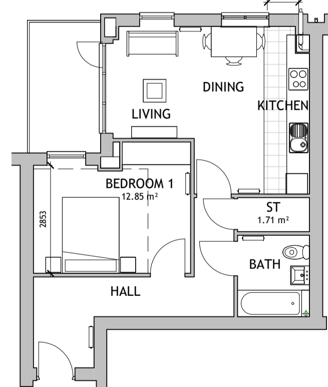
Flat P x 6 50.0m 2 1 : 100
