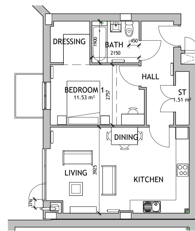
Flat N x 6 53.8m 2 1 : 100
