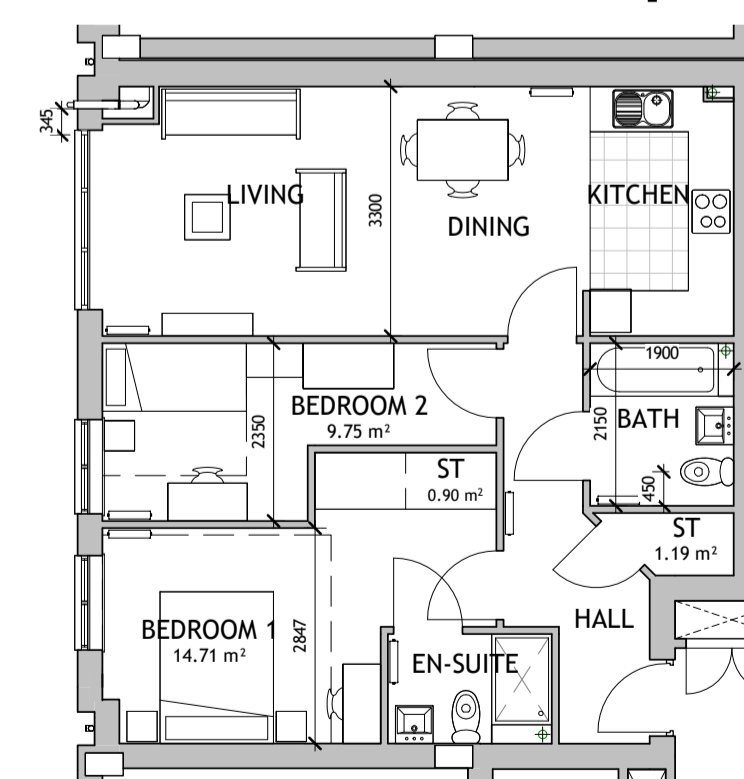
Flat R - Ensuite x 6 69.9m 2 1 : 100
