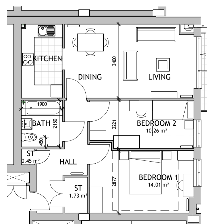
Flat R x 6 67.3m 2 1 : 100
