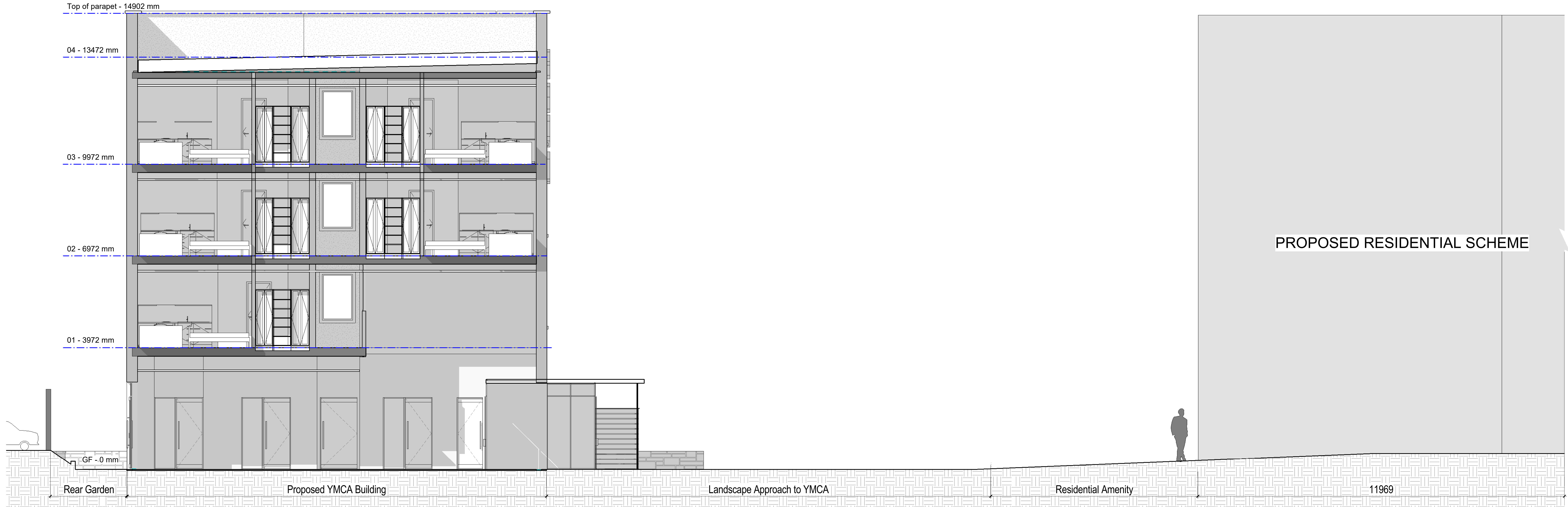
1 P116 - Hostel Sections A 1 : 50
