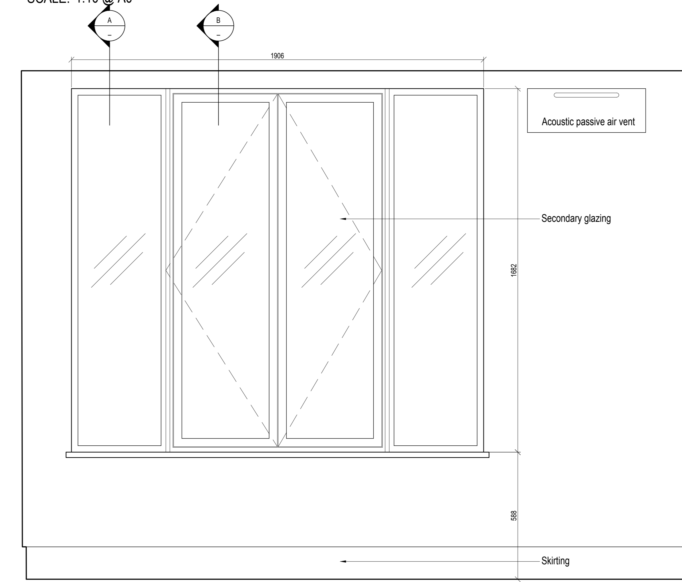
INTERNAL ELEVATION SCALE: 1:10 @ A0
