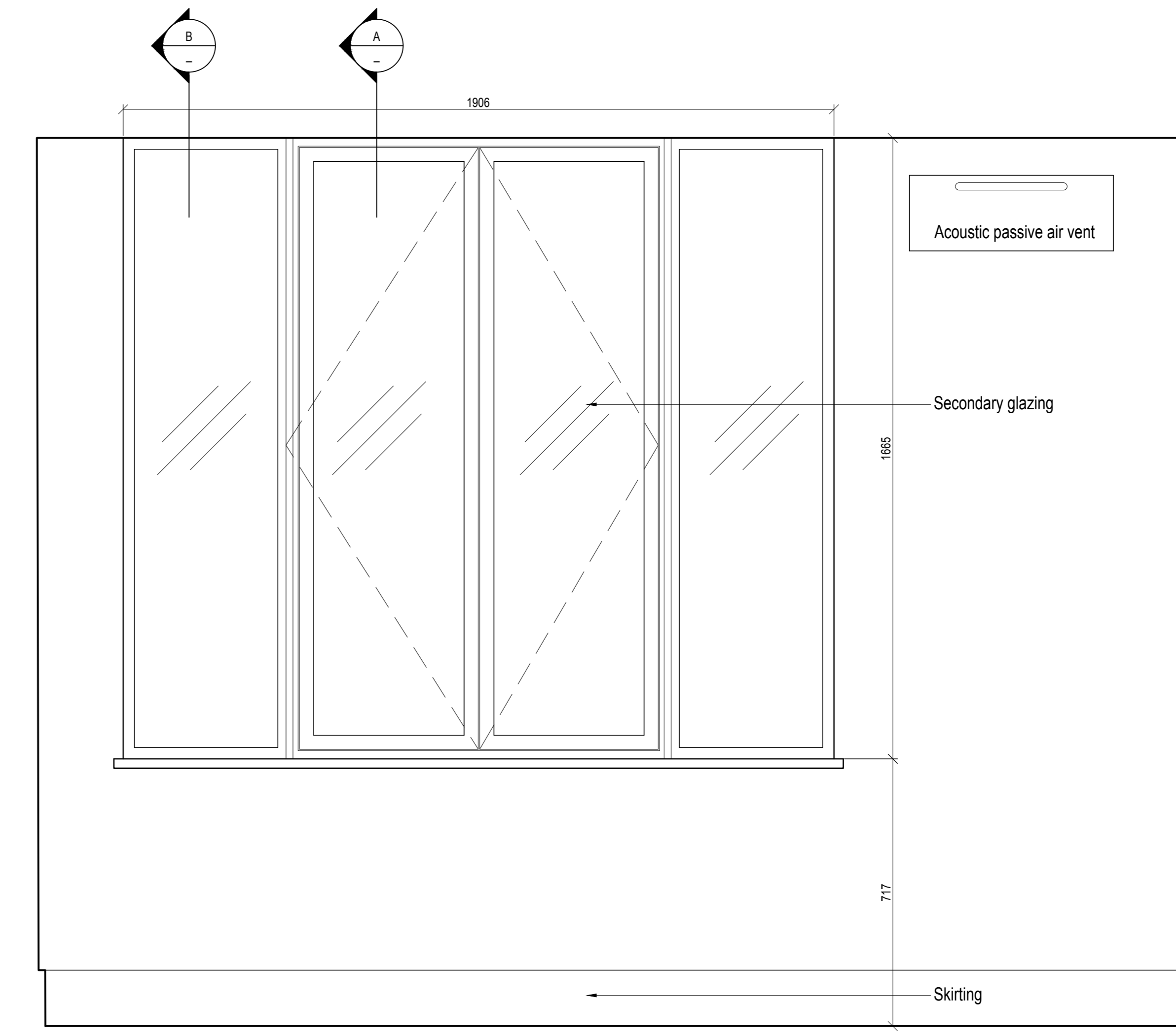
INTERNAL ELEVATION SCALE: 1:10 @ A0
