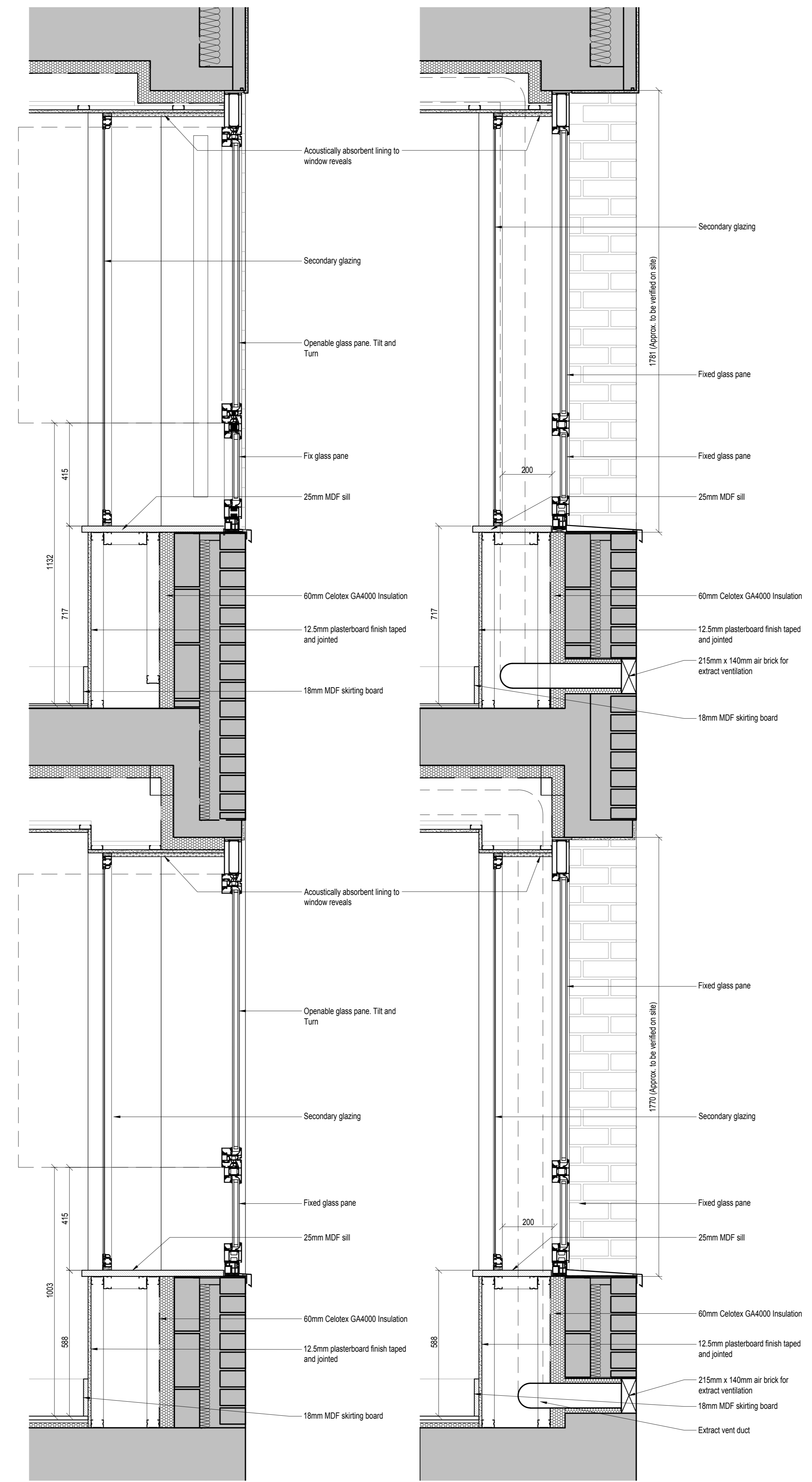
SECTION A SCALE: 1:10 @ A0 SECTION B SCALE: 1:10 @ A0
