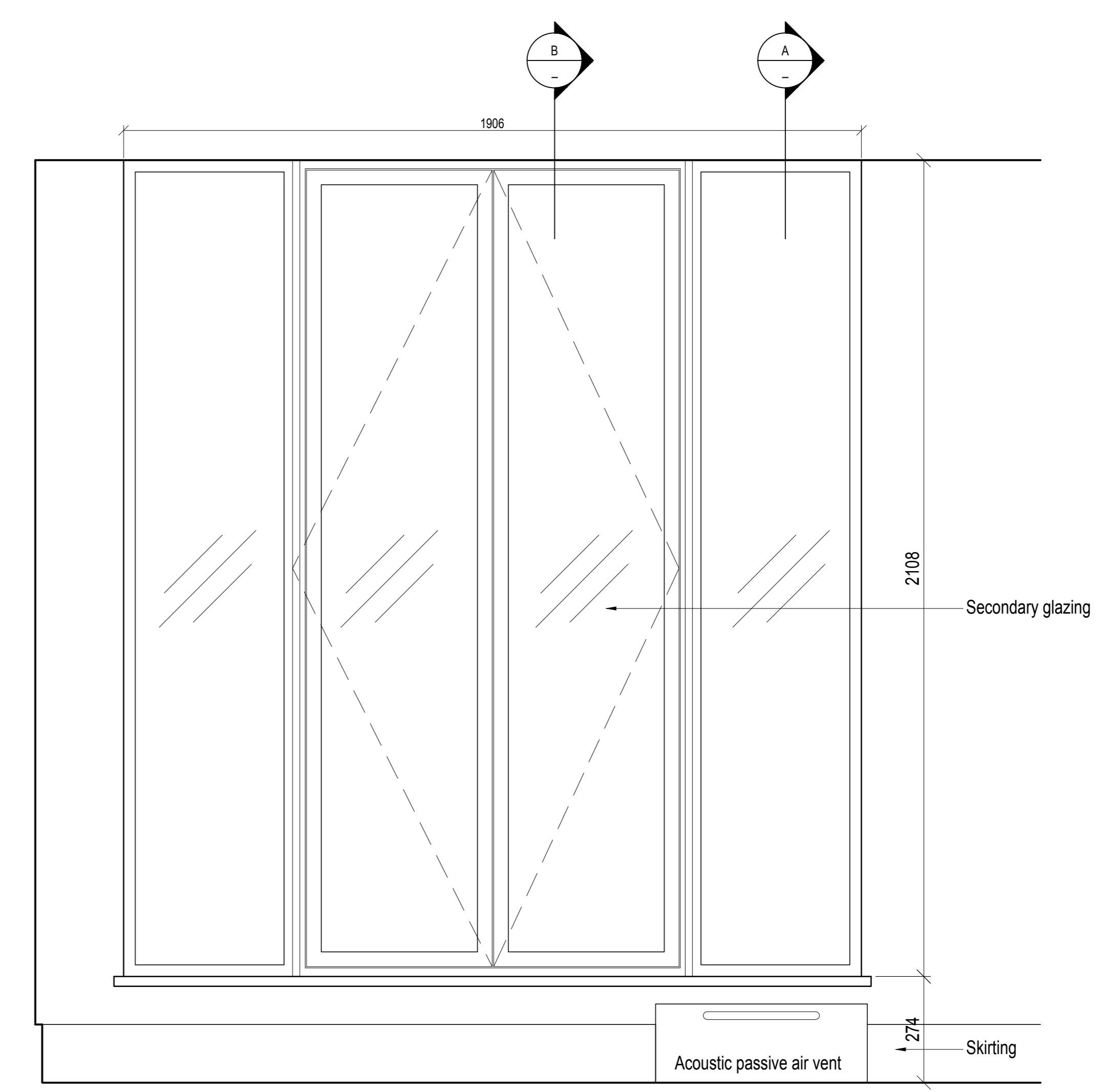
INTERNAL ELEVATION SCALE: 1:10 @ A0
