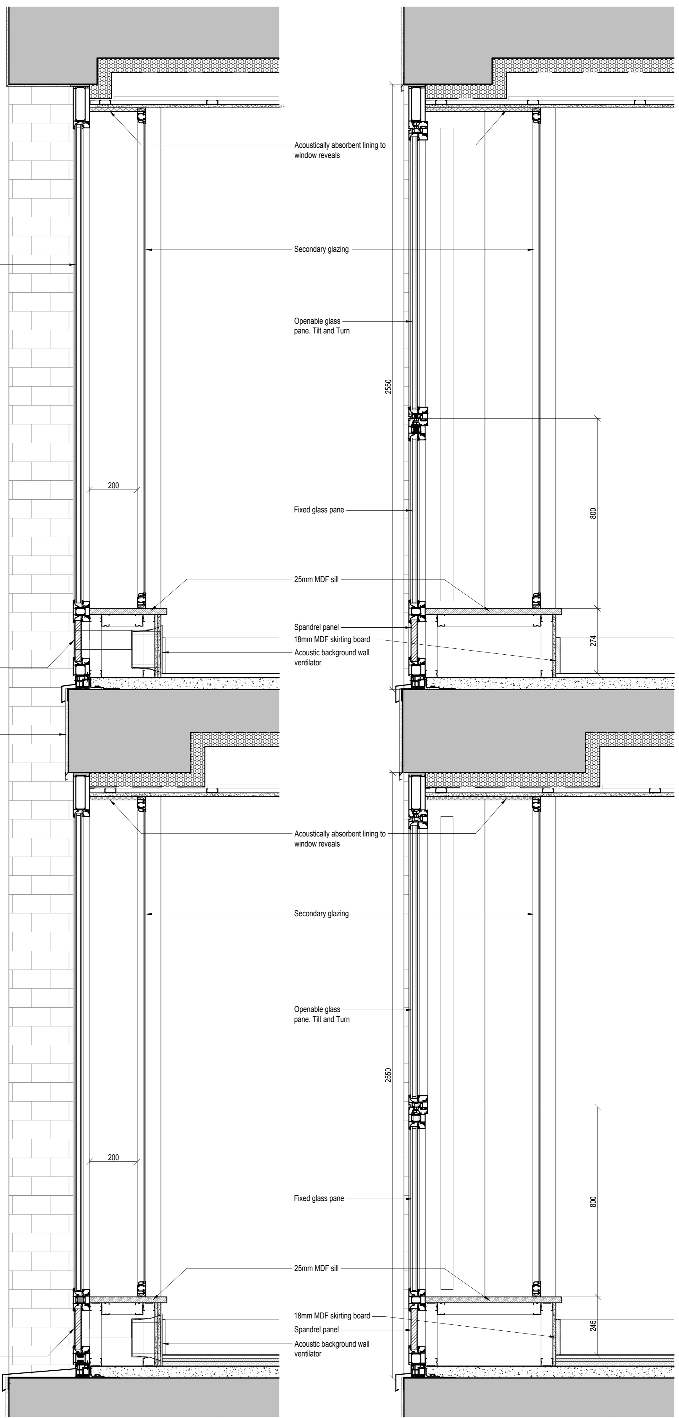
SECTION A SCALE: 1:10 @ A0
