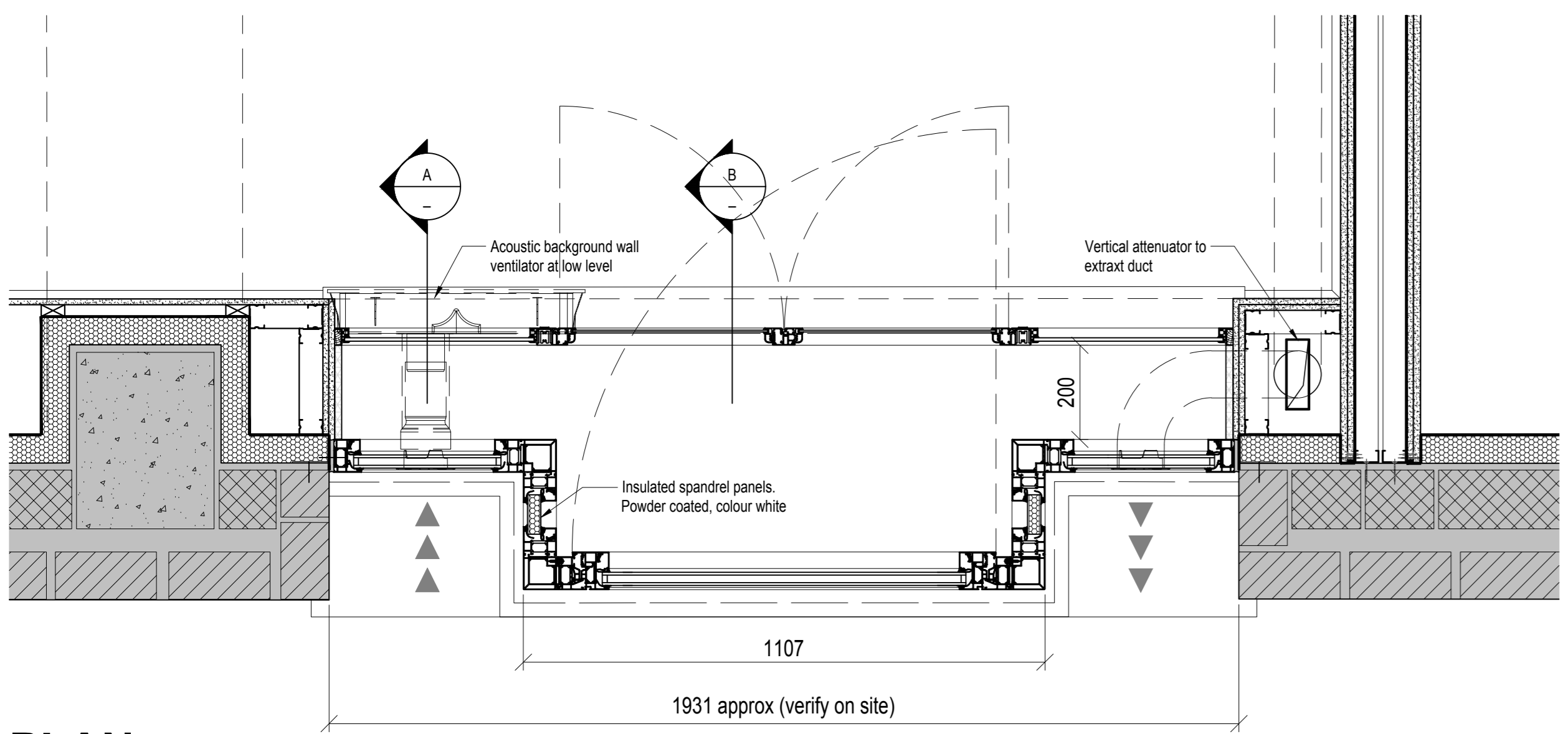
PLAN SCALE: 1:10 @ A0
