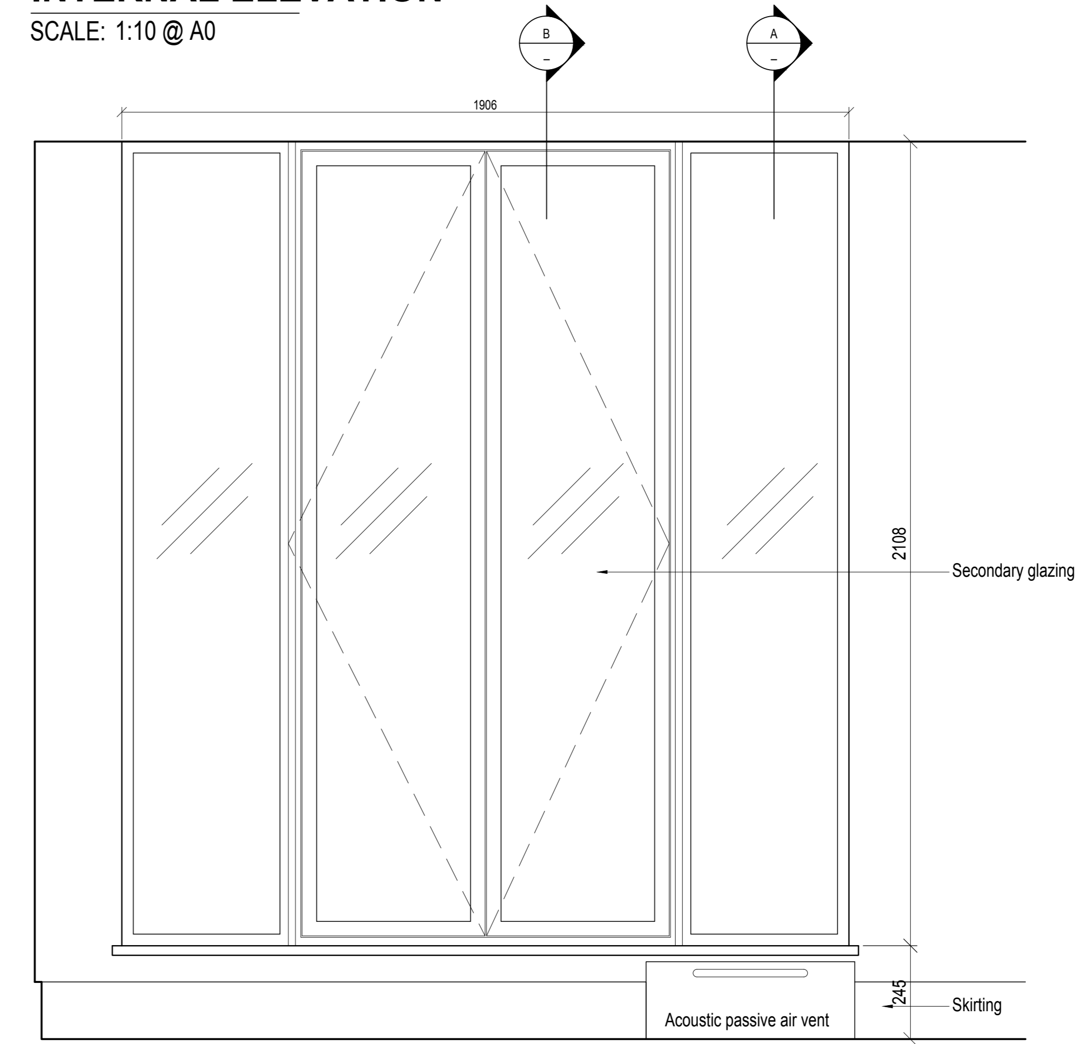
INTERNAL ELEVATION SCALE: 1:10 @ A0
