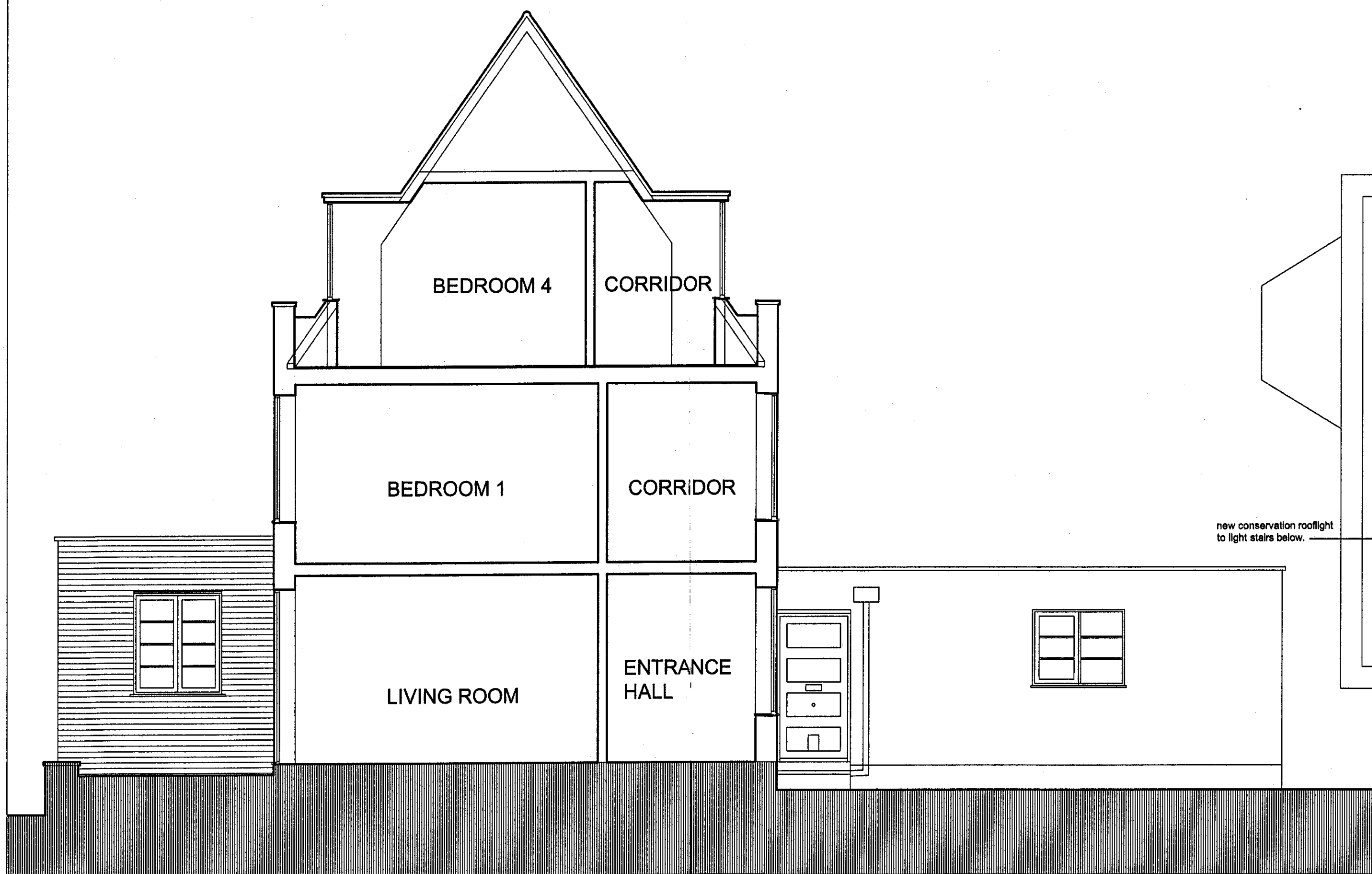
SECTION A-A
