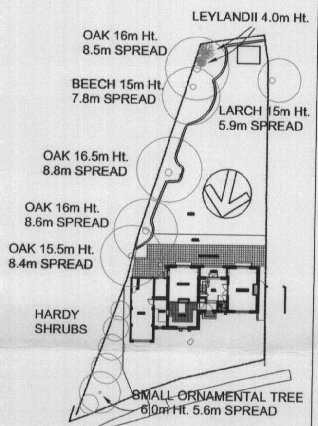
SITE PLAN 1:500
