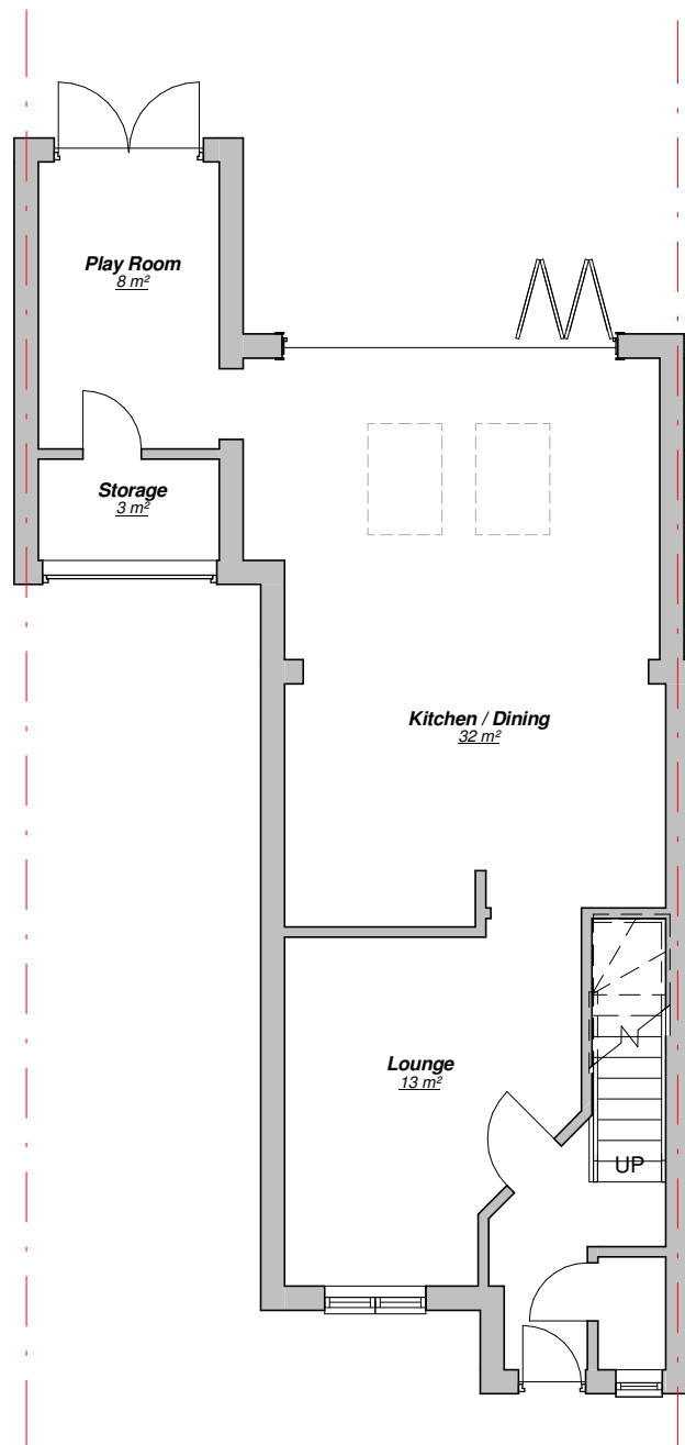
GF Lvl 1 : 100
