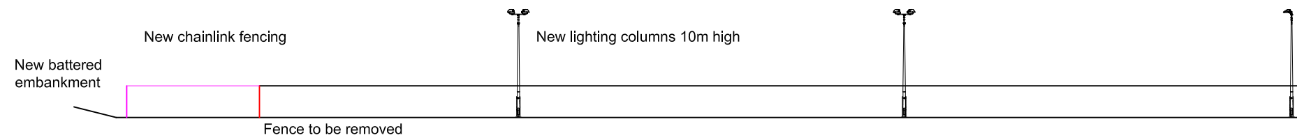
AA LONGITUDINAL SECTION SCALE: 1:500
