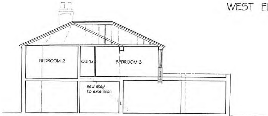
BASIC SECTION No:4
