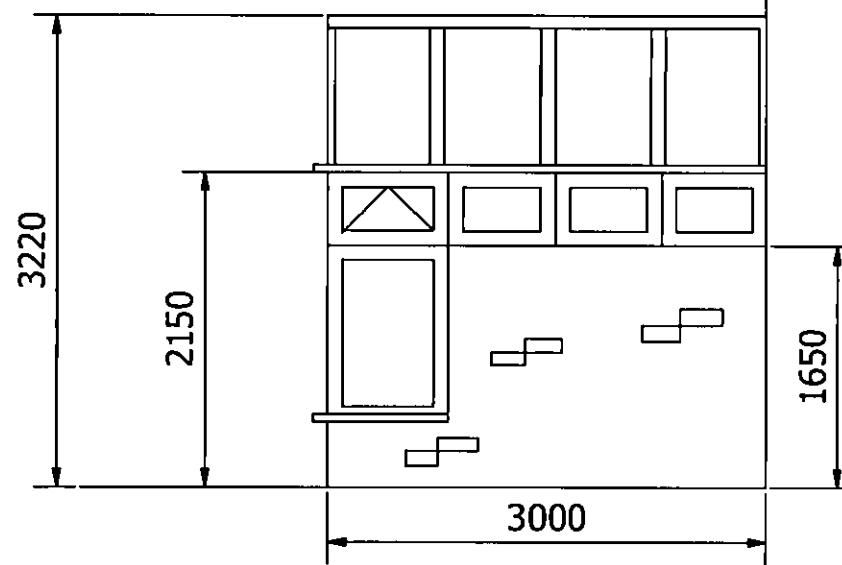
RIGHT ELEVATION
