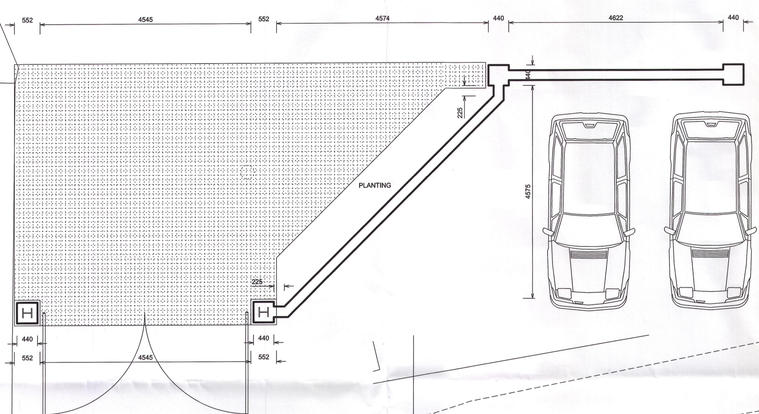
PLAN 1:50
