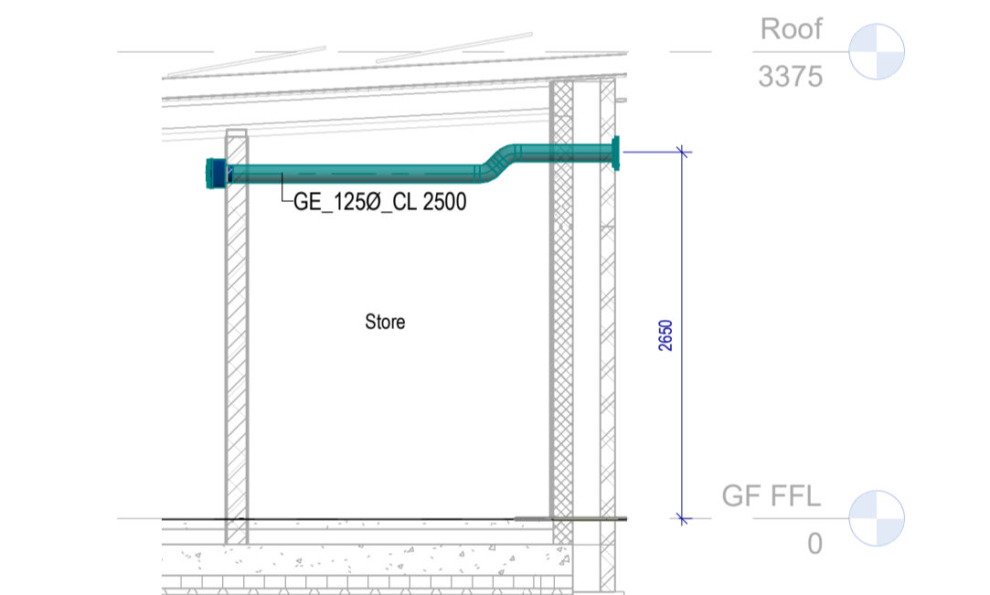
4 Section_Store 1:50
