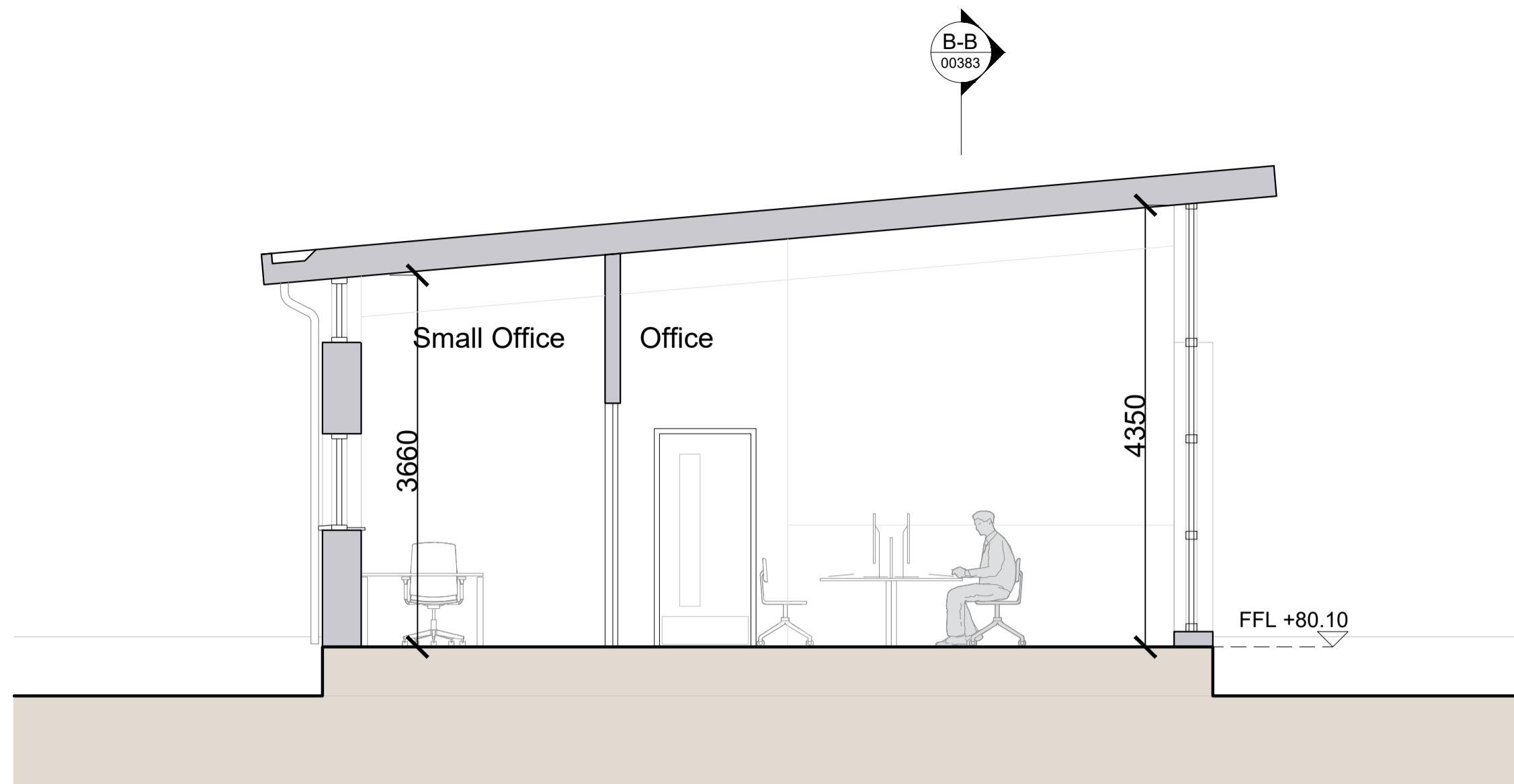
Section A-A
