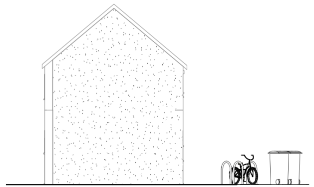
West. 1 : 100
