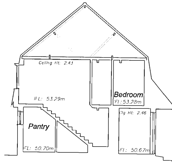
Datum: 50.00m. Section A - A.
