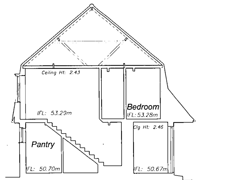
Datum: 50.00m. Section A - A.
