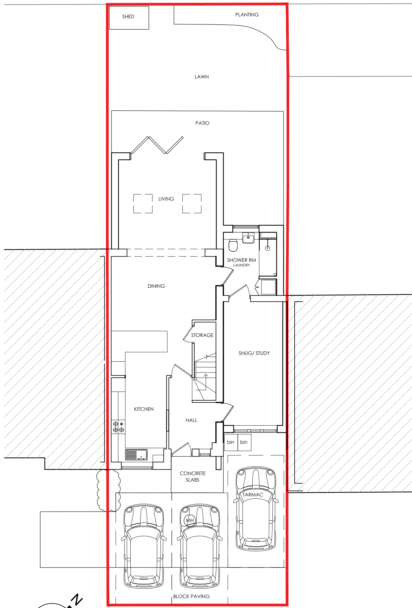
SITE PLAN 1:100
