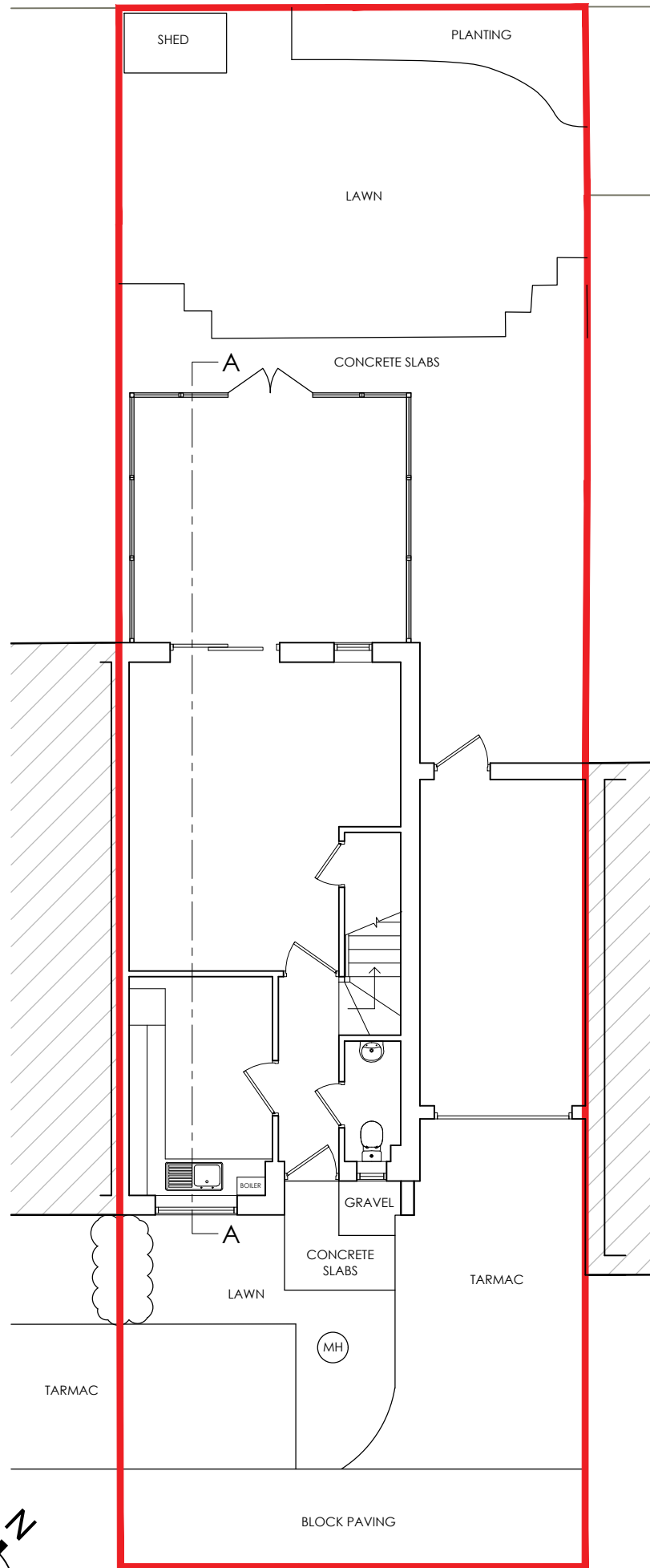
SITE PLAN 1:100
