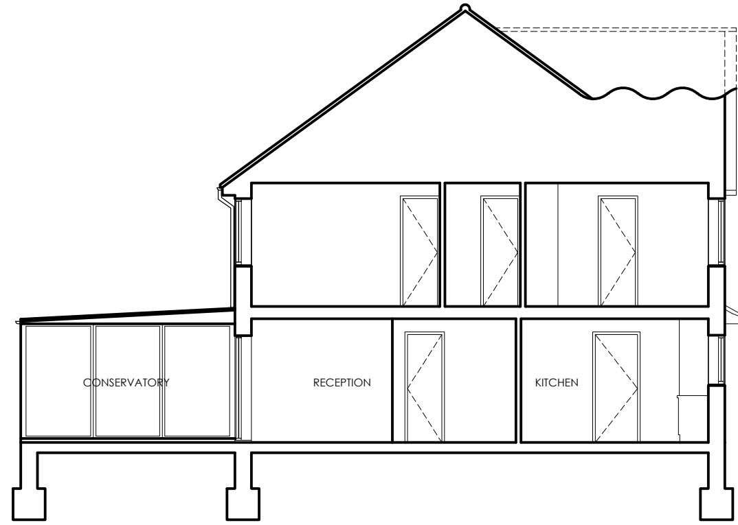
SECTION A-A 1:100
