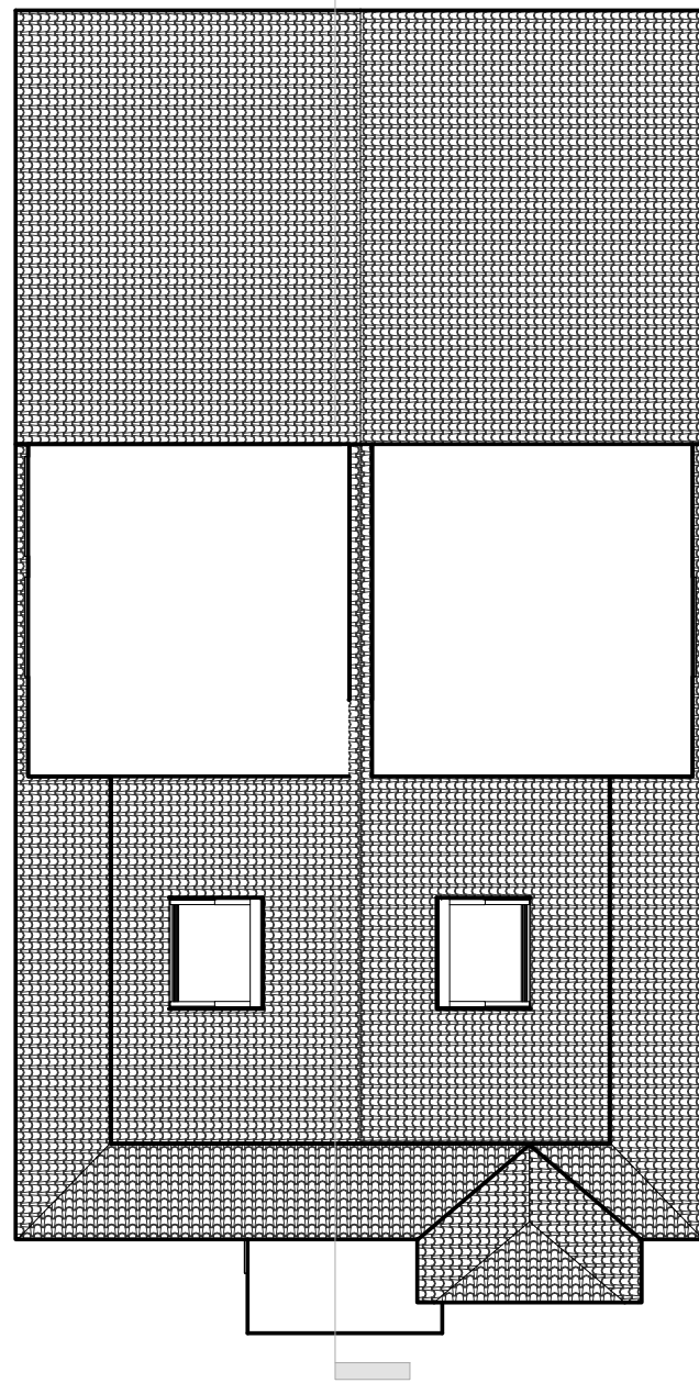
03. RL Existing 1 : 100
