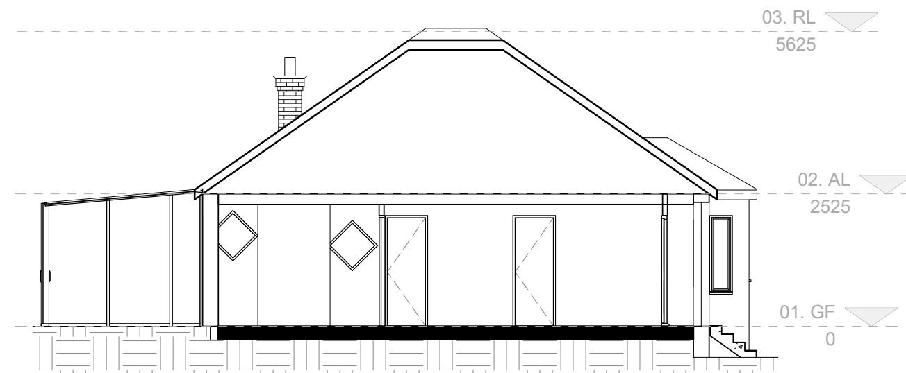
Section Existing 1 : 100
