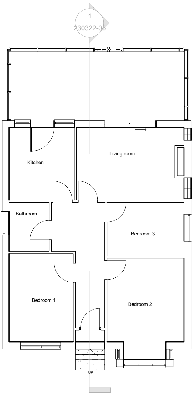
01. GF Existing 1 : 100
