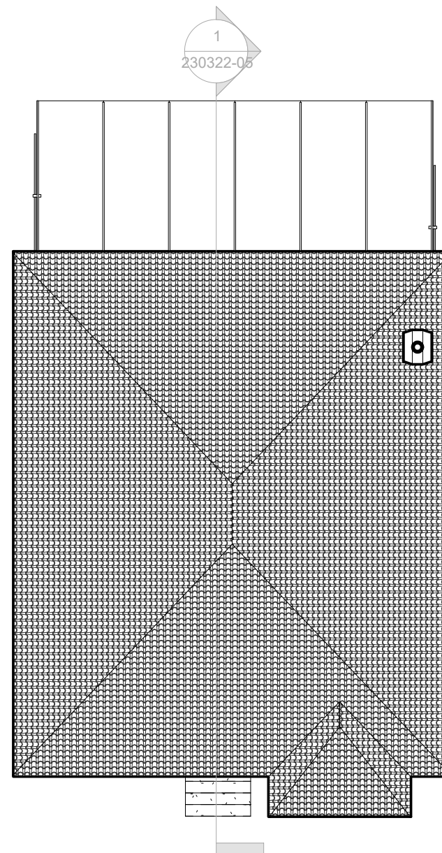
03. RL Existing 1 : 100
