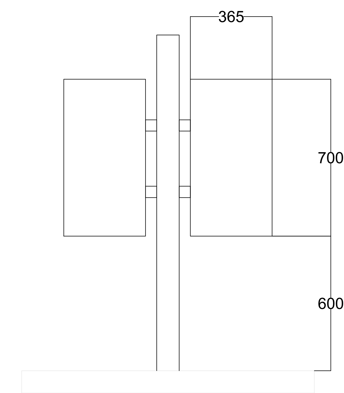
ELEVATION - END
