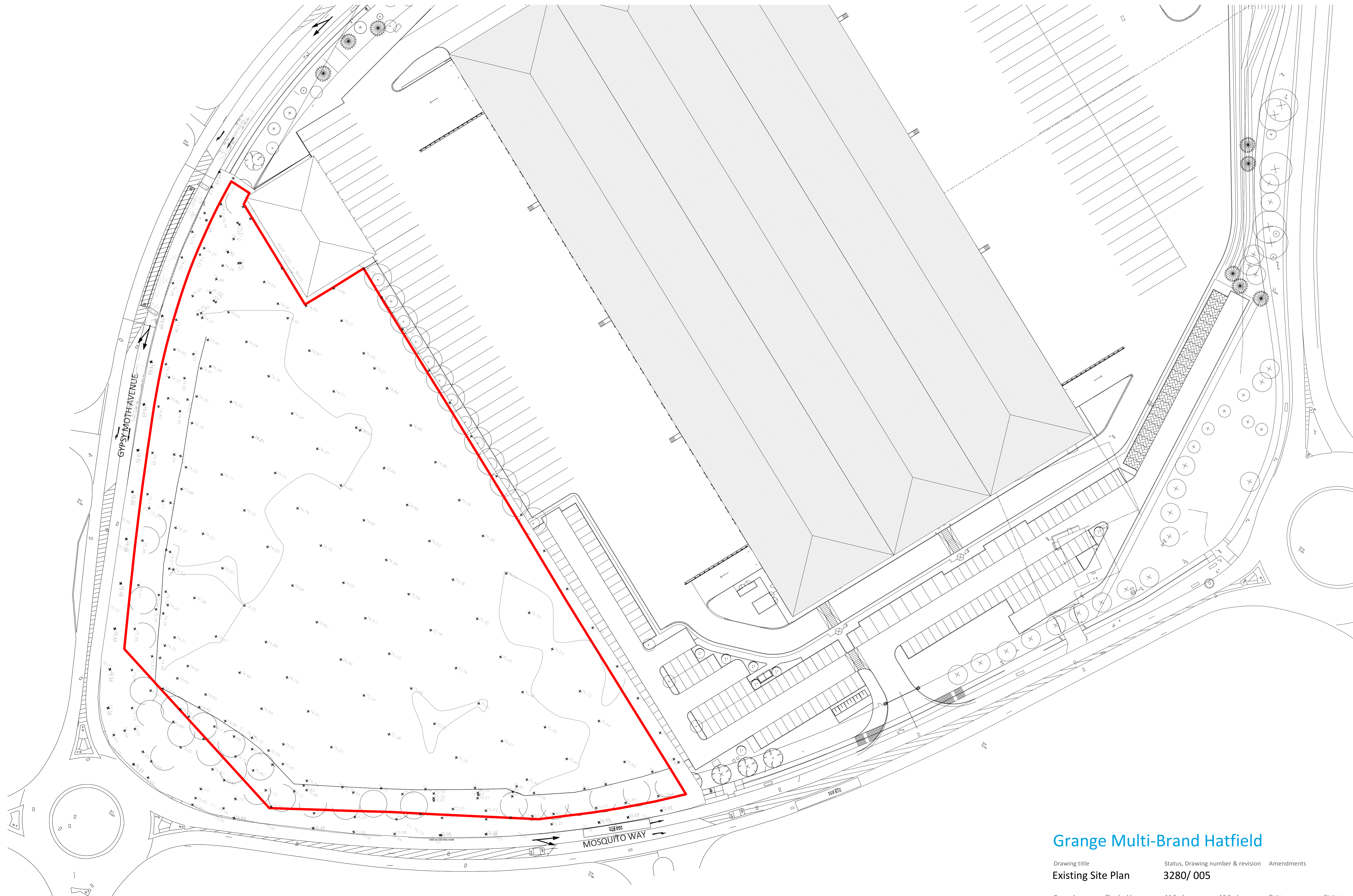
1 Existing Site Plan 1 : 500
