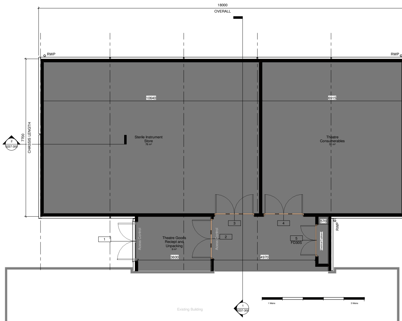
1 GF FFL (Partition Layout) 1 : 50
