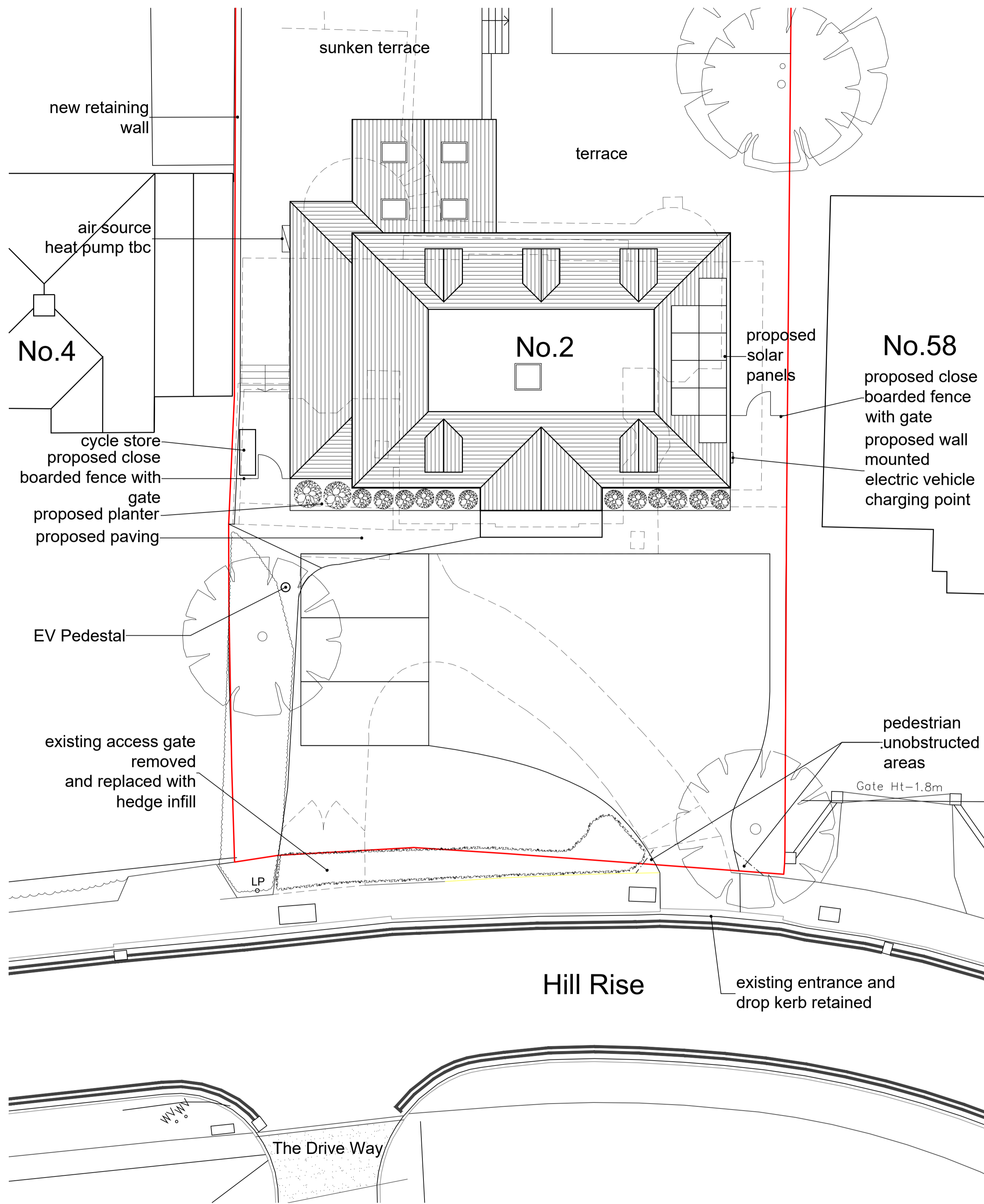
Site Plan 1:100 Scale
