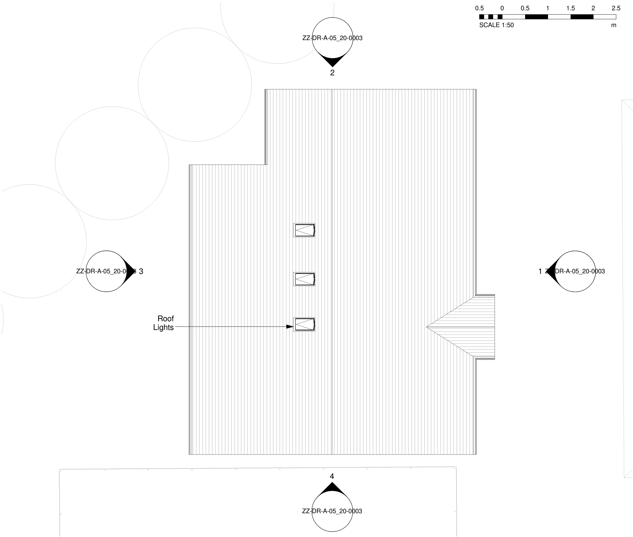
1 Roof Plan 1 : 100
