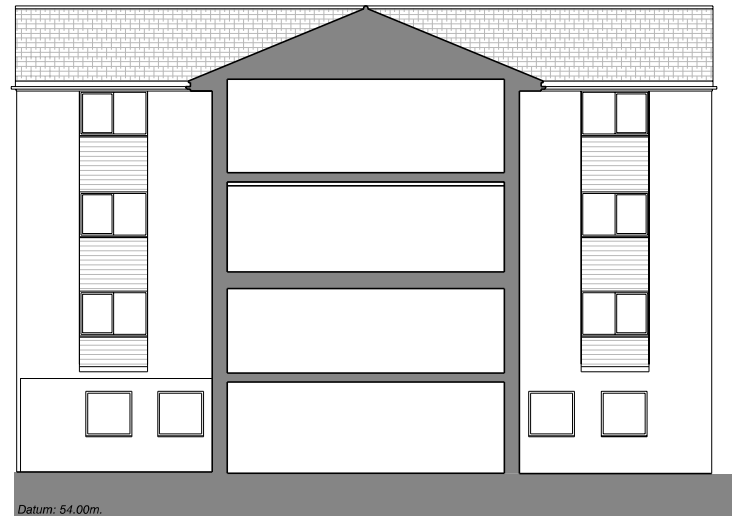
01 Elevation 4 1:200@A3
