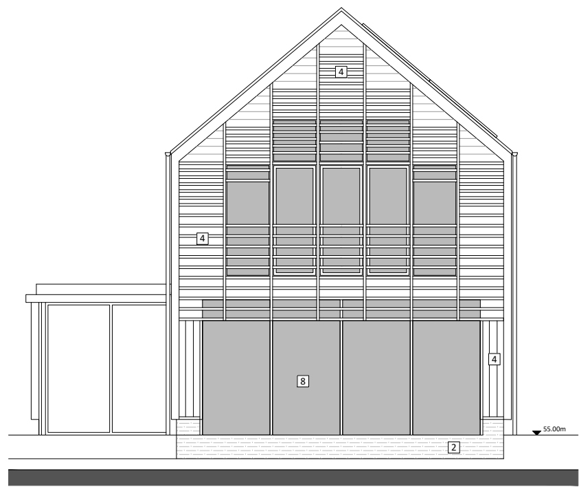
LH SIDE (SW) ELEVATION
