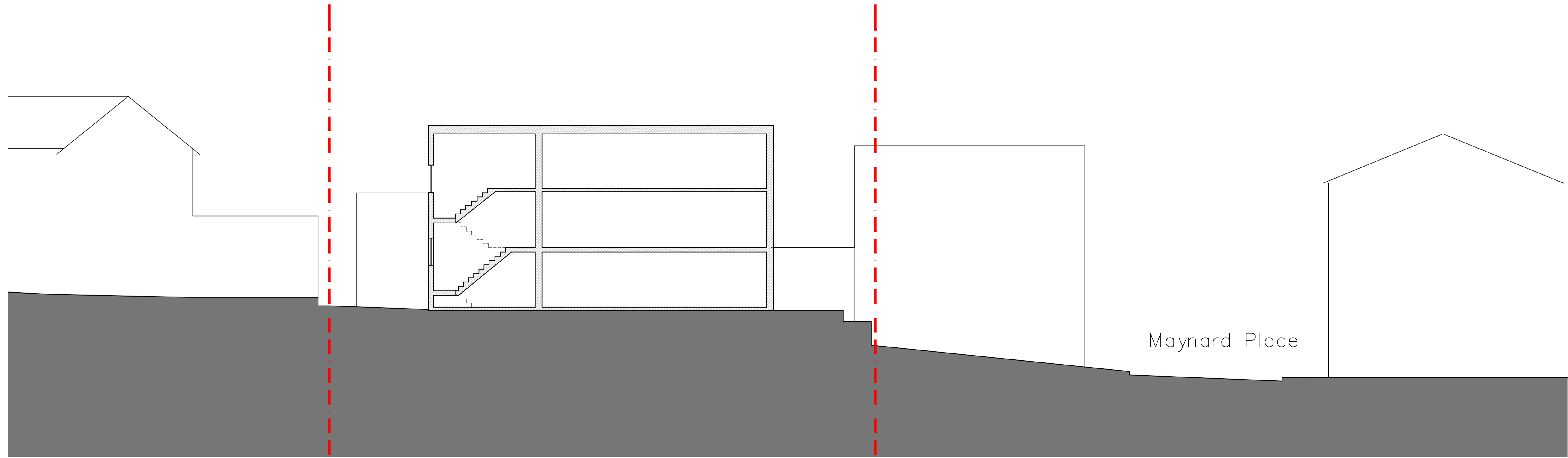
Existing Section A-A 1:100 @A1 / 1:200 @A3
