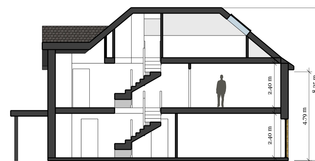
SECTION B-B scale: 1:100 J | 002
