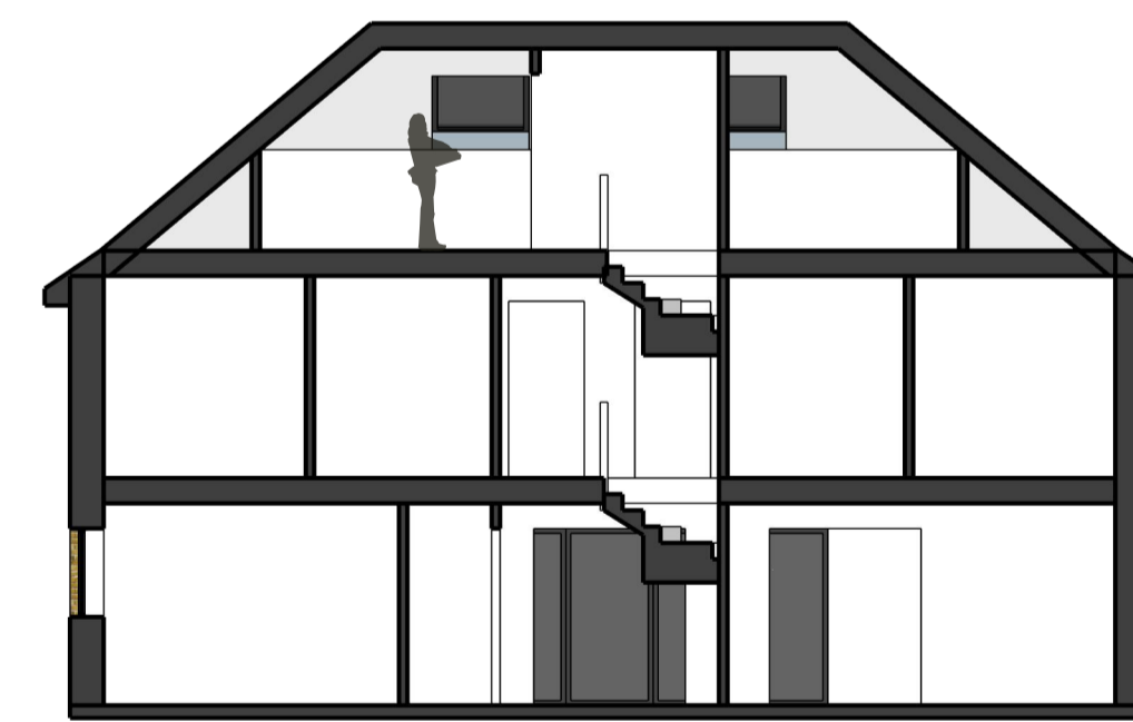
SECTION A-A scale: 1:100 I | 002
